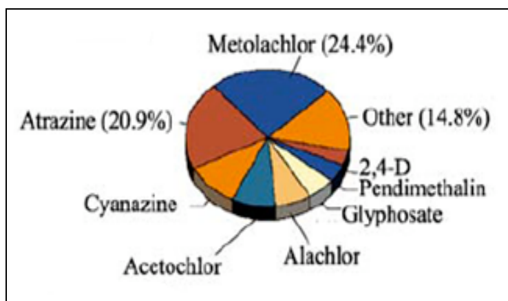
Figure 23. Pesticide usage in Lake Erie basin (Kanna, 2004).
